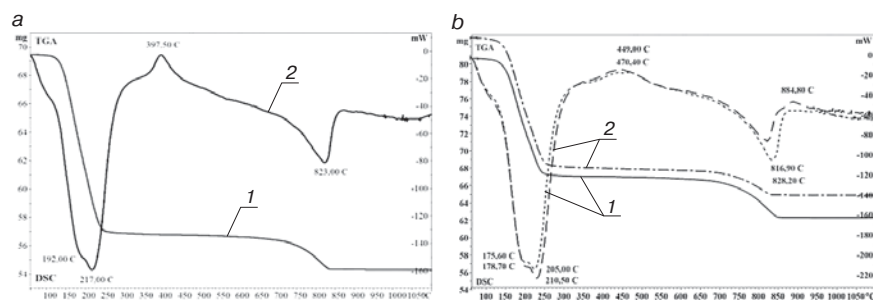
Рис. 8. ДТА анализ гипсовой матрицы: а – контрольный состав; б – составы с введением 5% цемента и 0,05% наносилики: 1 – без ультразвуковой активации; 2 – после активации ультразвуком
