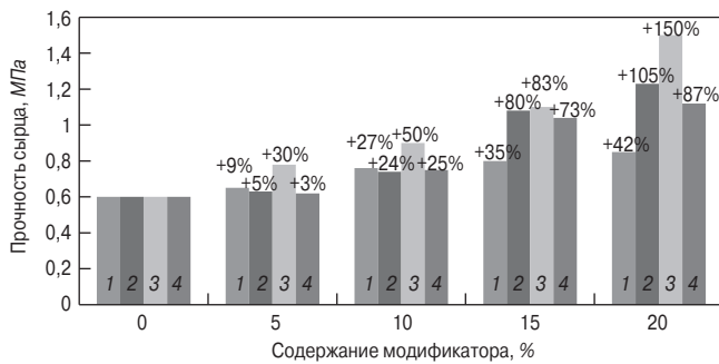
Рис. 1. Прочность сырца в зависимости от вида и содержания минерального модификатора: 1 – кварцевый песок; 2 – гранит; 3 – опока; 4 – перлит
