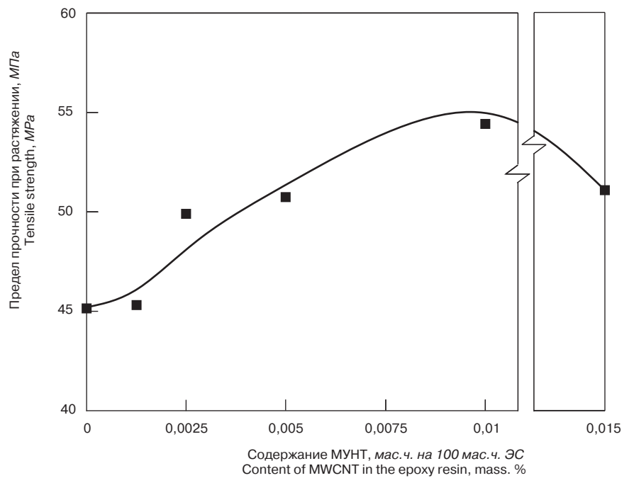
Рис. 1. Зависимость прочности при растяжении от содержания многослойных УНТ
