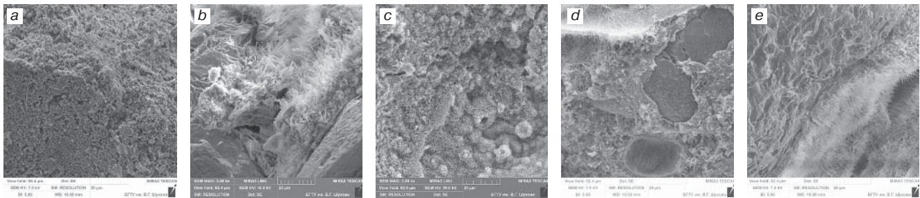
Рис. 3. Микроструктура автоклавированных силикатных изделий в зависимости от вида минерального модификатора: а – контроль; б – кварцевый песок; с – гранит; d – опока; e – перлит
