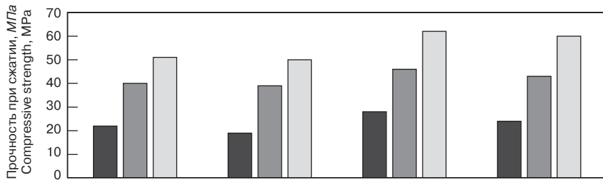
Рис. 1. Кинетика набора прочности портландцемента и композиционных вяжущих: 1 – исходный портландцемент; 2 – портландцемент + зола-уноса 30%; 3 – портландцемент + УНМ; 4 – портландцемент + зола-уноса 30% + УНМ: ■ – 2 сут; ■ – 7 сут; ■ – 28 сут
