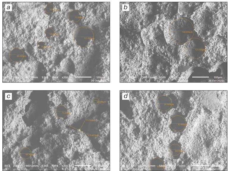
Рис. 3. Структура пористости газобетонов: а – ПЦ; б – ПЦ+ЗУ; с – ПЦ+УНМ; д – ПЦ+ЗУ+УНМ
