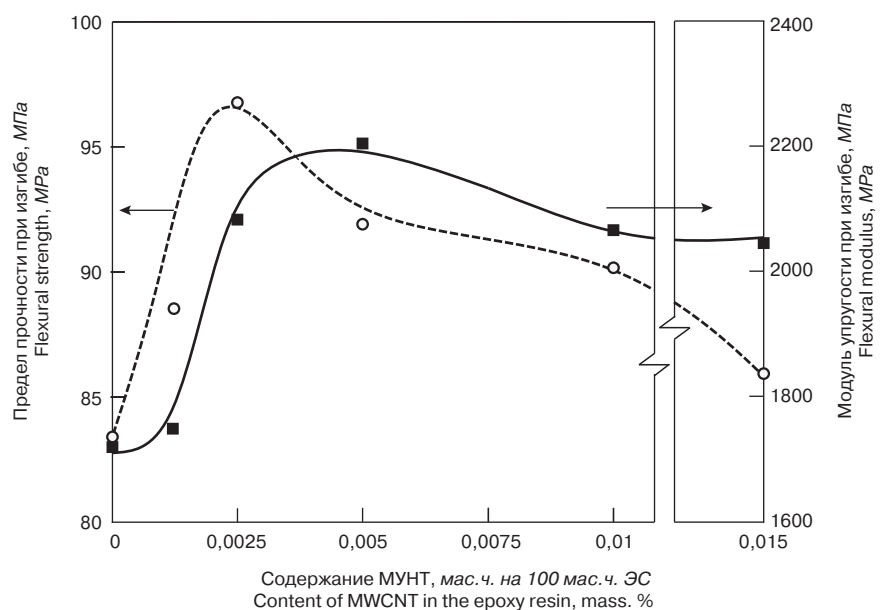
Рис. 2. Зависимости прочности и модуля упругости при изгибе от содержания многослойных УНТ
