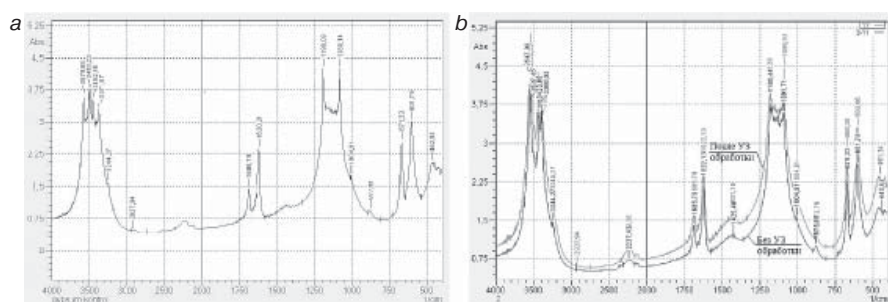
Рис. 7. ИК-спектры гипсовой матрицы: а – контрольный состав; б – составы с введением 5% цемента и 0,05% наносилики до и после ультразвуковой обработки
