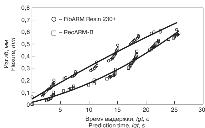
Рис. 4. Обобщенная кривая ползучести железобетонной балки, усиленной СВА на адгезиве RecARM-B и FibArm 230+
